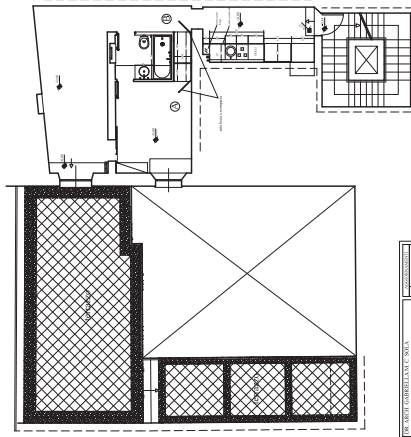
PIANTA - opp. 1:50
