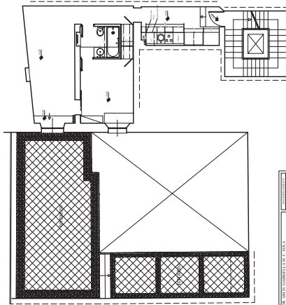
PIANTA - opp. 1:50
