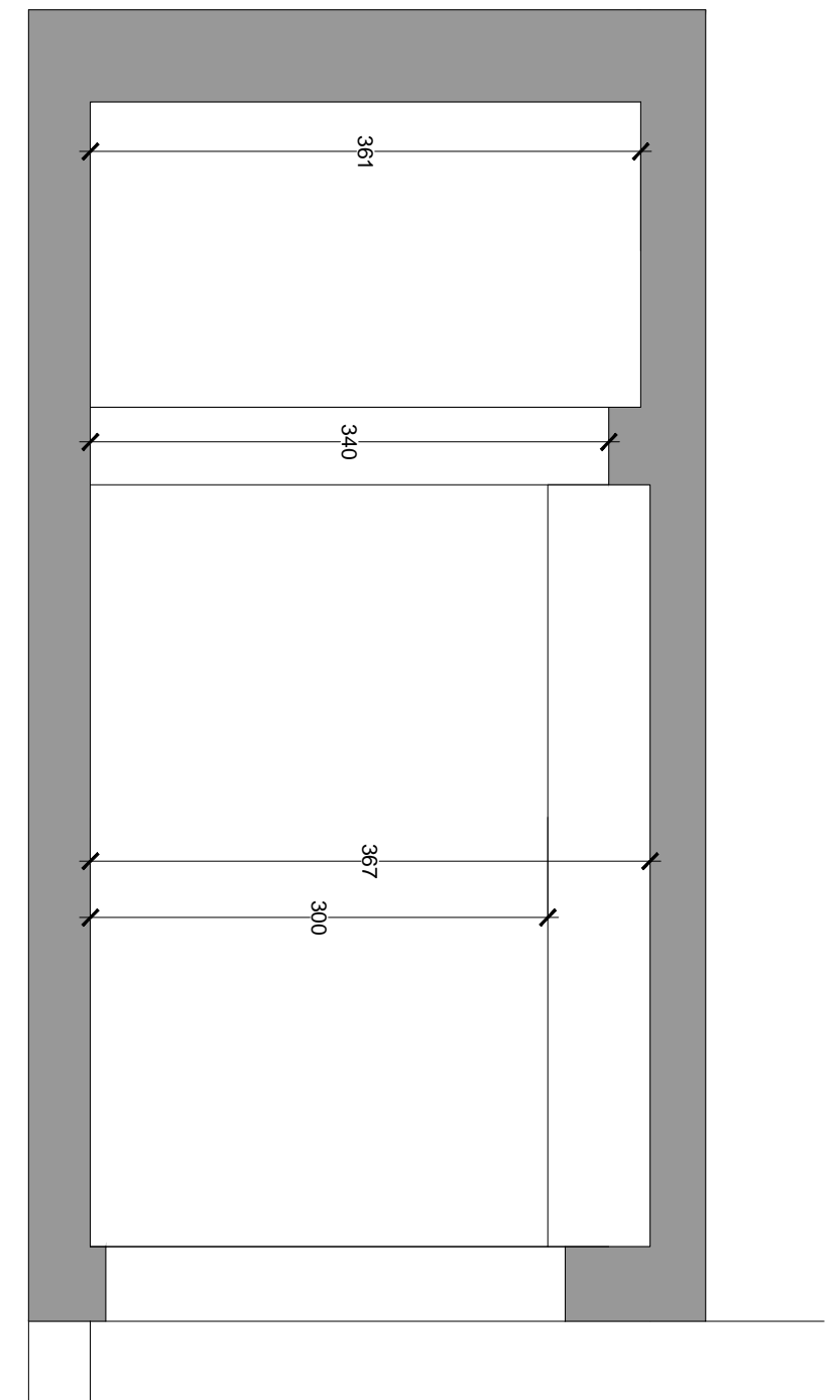
Sezione A.A Negozio
