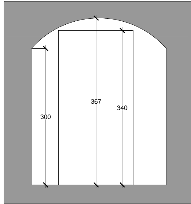
Sezione B.B Negozio
