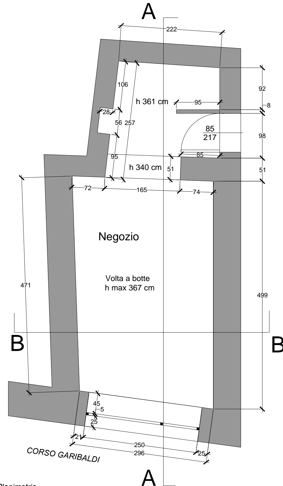
Planimetria Negozio - Piano Terra
